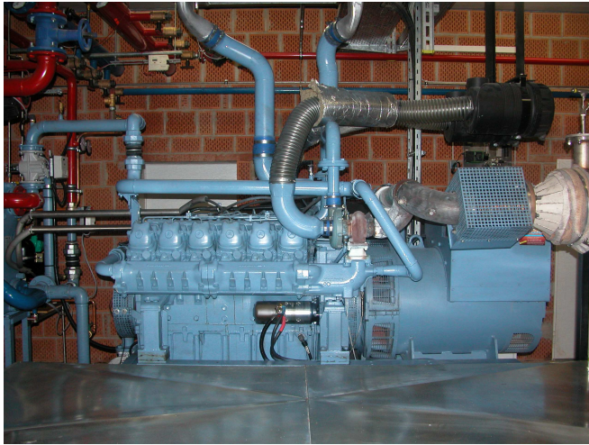
Pflanzenöl- BHKW der Gärtnerei Mayer mit einer Leistung von 300kW el
